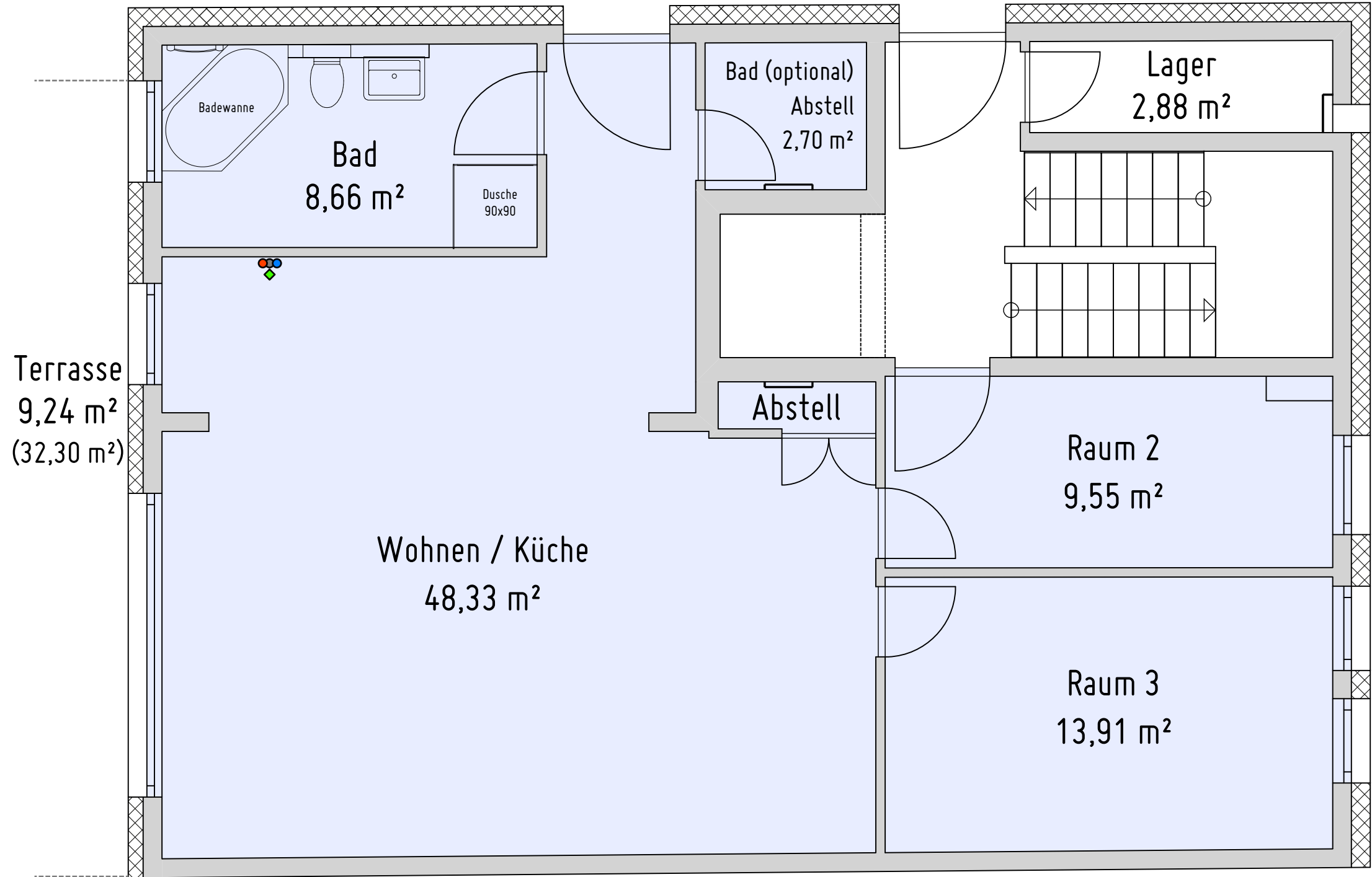
Erdgeschoss als 3-Zimmer-Wohnung
