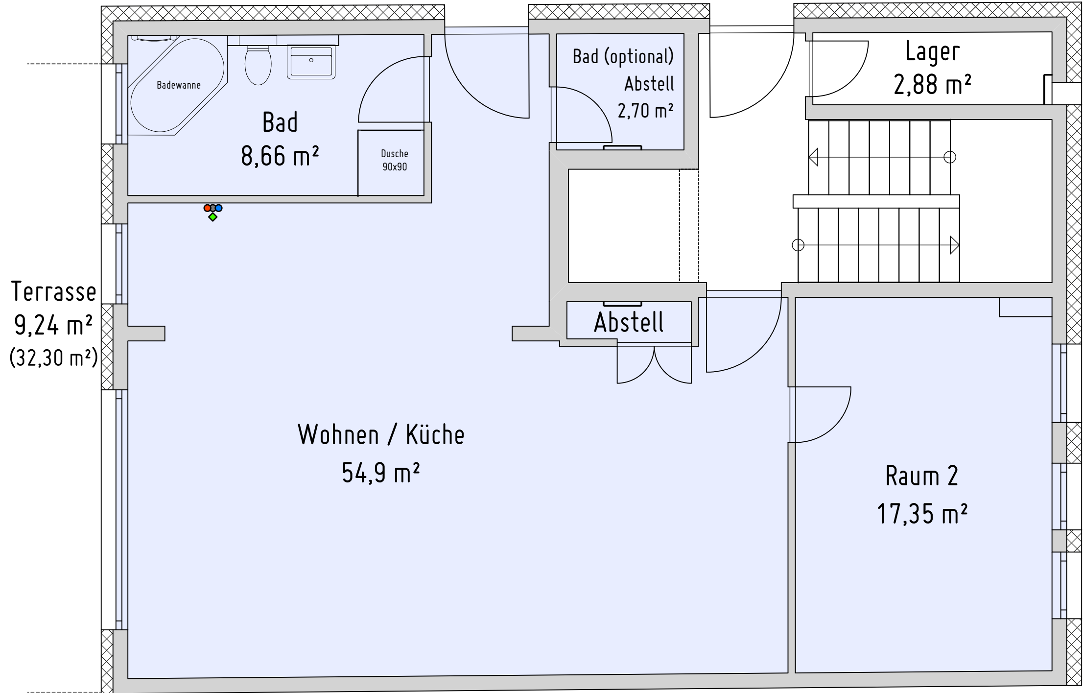
Erdgeschoss als 2-Zimmer-Wohnung
